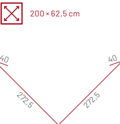
Rynna koszowa F11
