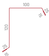
Wiatrownica boczną F02
