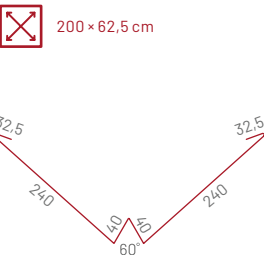
Rynna koszowa z mostkiem F12
