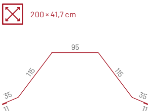
Obróbka kalenicy trapezowa płaska F27
