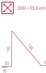
Bariera przeciwśniegowa F20
