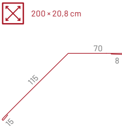
Obróbka nadrynnowa F09
