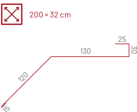
Obróbka nadrynnowa z nadbiciem F26
