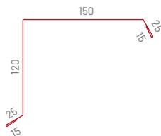
Wiatrownica boczną F02
