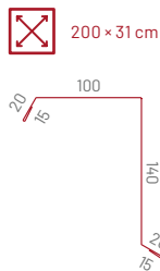
Wiatrownica nakrywająca z rynienką (komplet) F25
